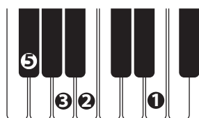
H7sus4
