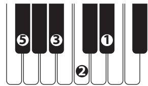
Cm7b5
