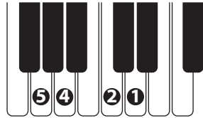
D7sus4
