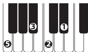
F7sus4
