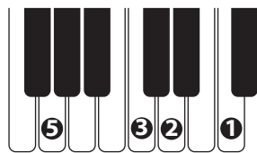
G7sus4
