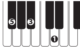
Daug (F#aug)
