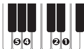
A7sus4
