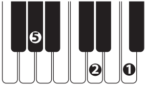
Ddim
