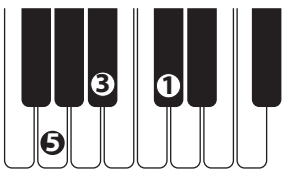
Gdim
