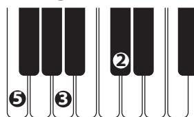
Faug
