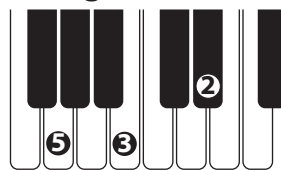
Gaug
