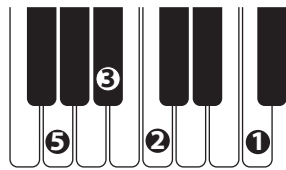
C7sus4
