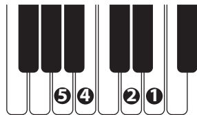
E7sus4
