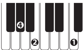
Fdim
